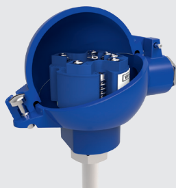
Insert de mesure avec transmetteur installé (ici : type T32)
