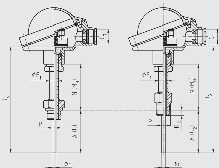
filetage parallèle
