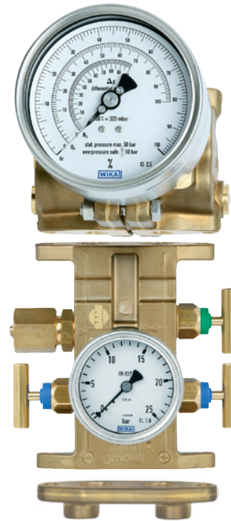
Fig. in alto: manometro differenziale modello 712.15.100
