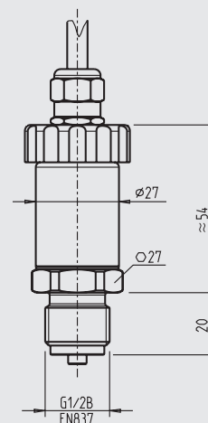
mit Kabelausgang, Standard gang
