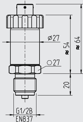
mit Bajonettstecker (6-polig)
