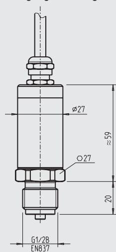
mit Kabelausgang, nicht abgleichbar
