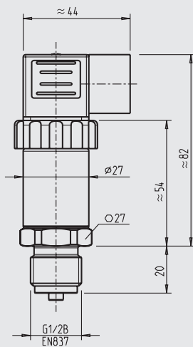
mit Winkelstecker DIN 175301-803 mit 1/2 NPT
