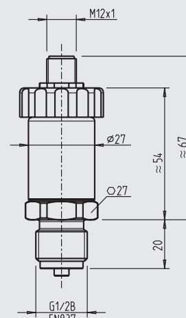
mit Rundstecker M12 x 1 (4-polig)
