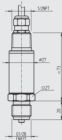
mit 1/2 NPT Conduit außen, mit Kabelausgang
