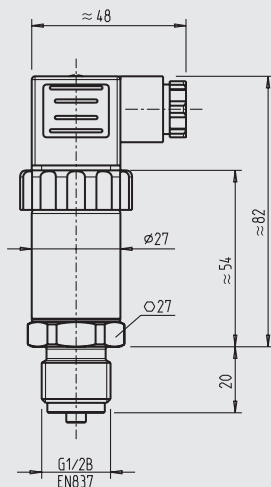
mit Winkelstecker DIN 175301-803 A
